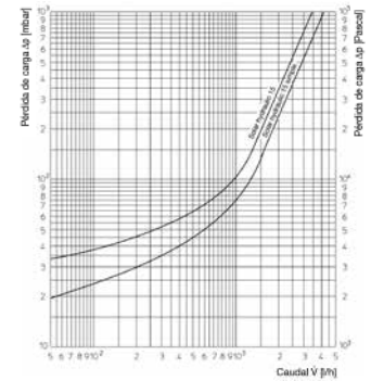
Pérdida de carga del grupo hidráulico
