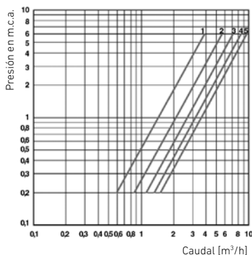
Pérdida de carga
