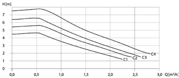
Curva característica del circulador
